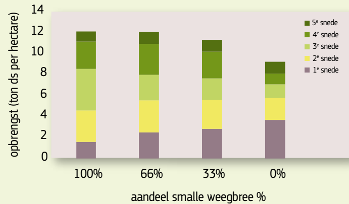
Figuur 3.3: Cumulatieve droge stof opbrengst van smalle weegbree, Engels raai-gras en hun mengsels in 2018 (1 e jaar na inzaai op veeggrond).
